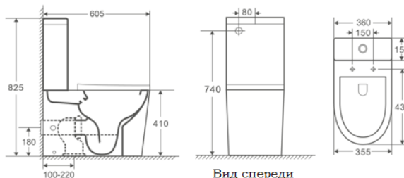
Вид спереди
